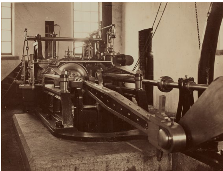
Machines in het Beijerinckgemaal (NL-RtSA_4187_XXXIII-80-02-6)
